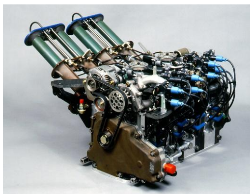
R26B 4-rotorowy silnik z Mazdy 787B
